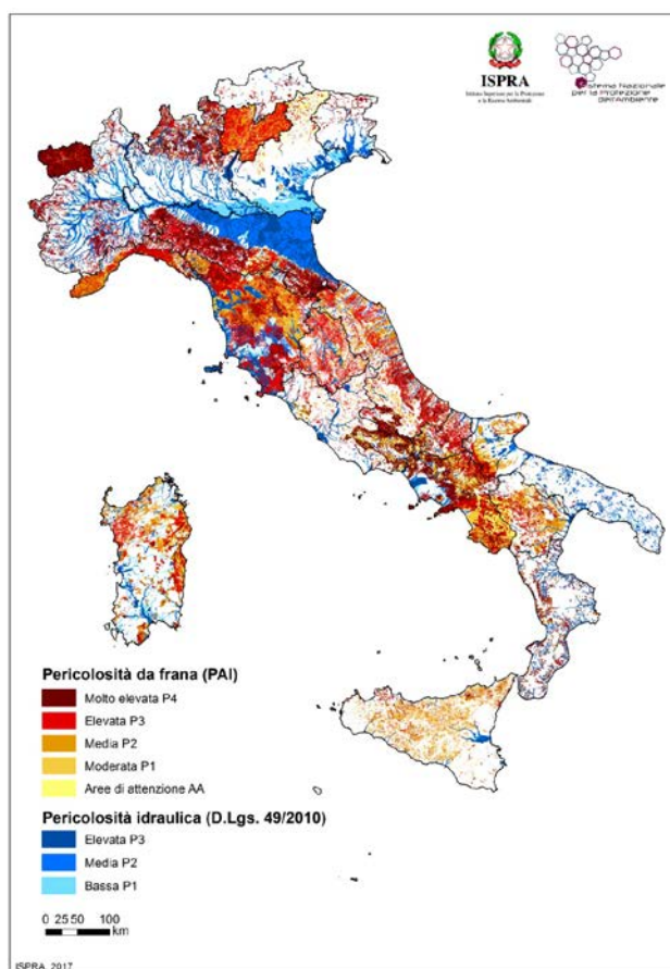
Figura 3.1 - Aree a pericolosità da frana (PAI) e idraulica (Scenari D.Lgs. 49/2010) – Mosaicature 2017
