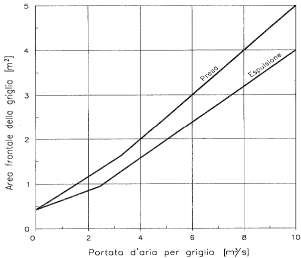
Figura J.9 - Diagramma per la scelta delle griglie (Fonte: miniguide Aicarr 2010)
