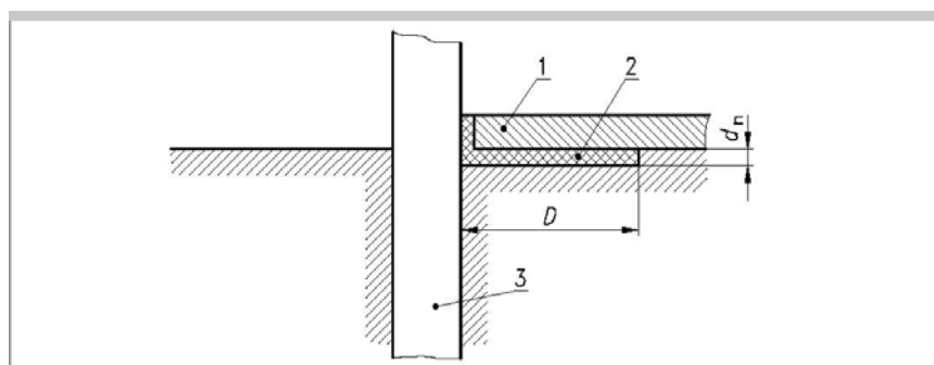
Figura B. 2 - Isolamento perimetrale orizzontale
