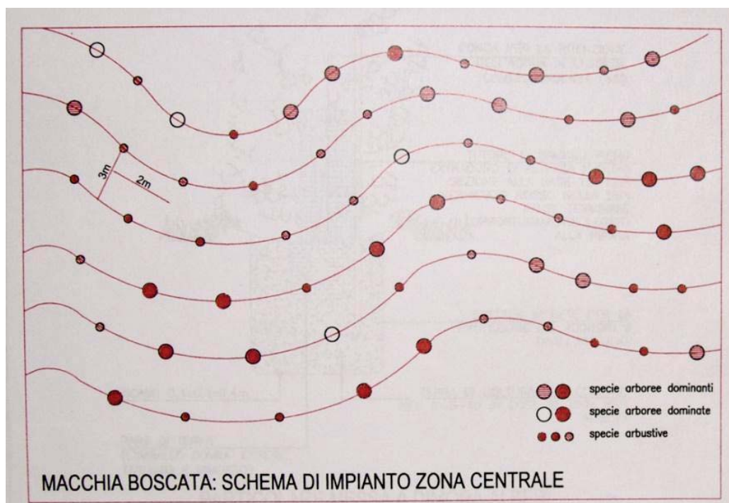
Fig. 6 Esempio di schema d'impianto a linee curve parallele
