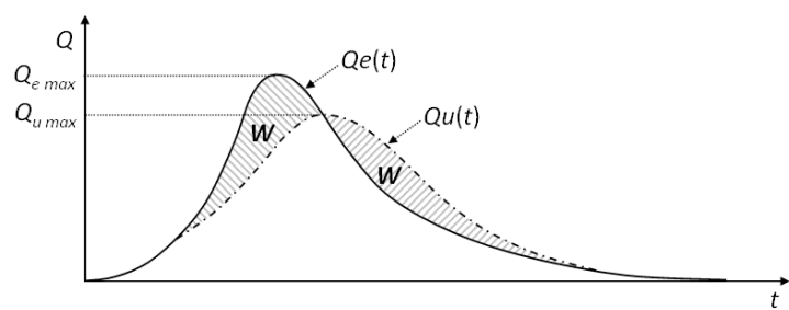
Figura 2 - Rappresentazione schematica del processo di laminazione di un invasivo in linea
